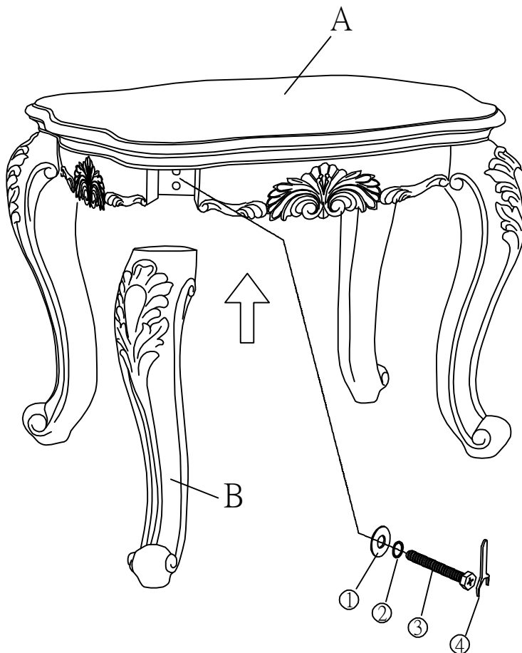
B:LEGS*4PCS
